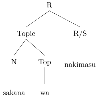
図 2: 日本語文法 1 による 'sakana wa nakimasu' の分析
